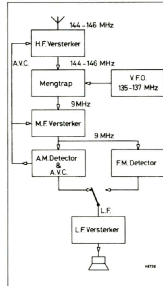
VERON SP81 2m ontvanger
