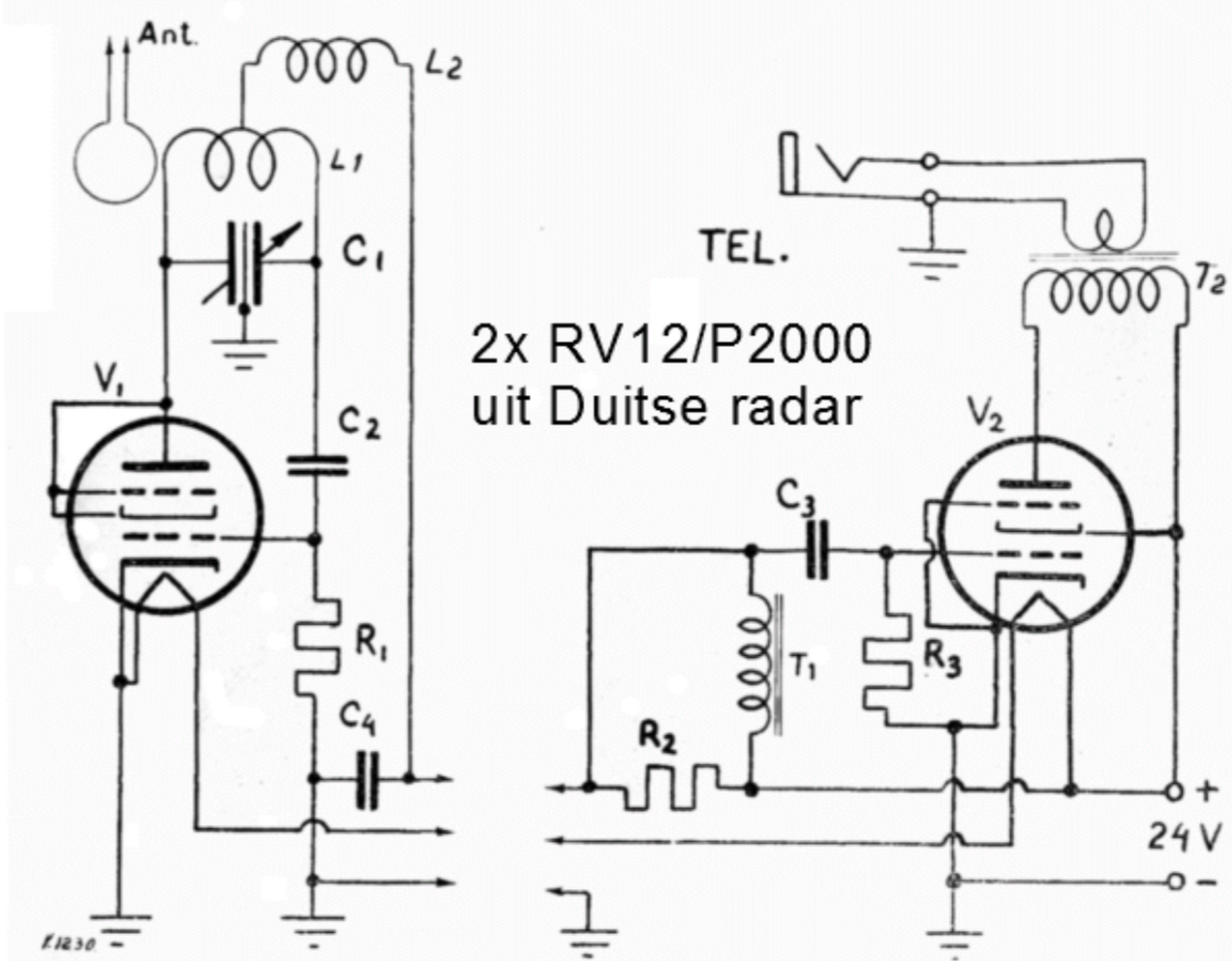
Peilen op 2 meter! Met recht kan hier worden gesproken van een dubbel-loop's jachtgeweer! (Foto Hackmann)
