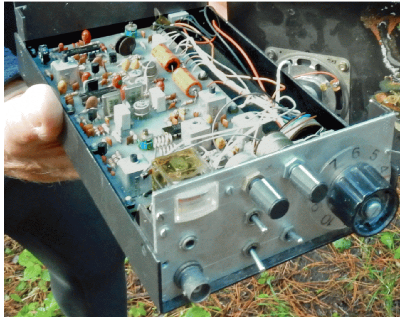
VERON SP81 2m ontvanger
