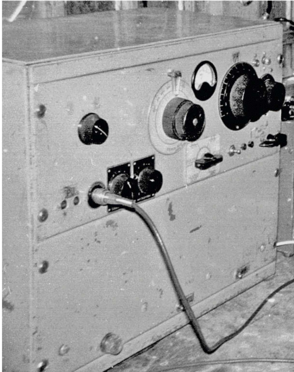
Vossenjachtzender met Ronette microfoon in gebruik vanaf 1948, door PA0KI c.s.
